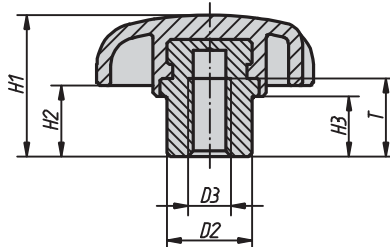
Form K mit Gewindebuchse
