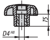
Form H mit Passbuchse
