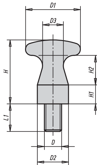
Flacher Knopf mit Außengewinde
