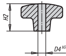
Form B durchgehende Bohrung
