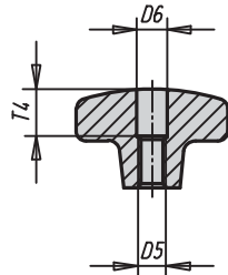
Form D Gewinde aufgebohrt
