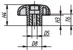
Form K mit Gewindebuchse mit Deckel
