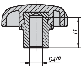
Form H Buchse mit Sackloch
