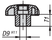
Form G ohne Buchse
