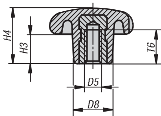
Form K mit Gewindebuchse
