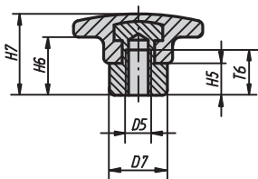
Form E mit vorstehender Stahlbuchse
