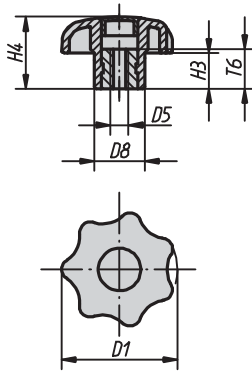
Form K mit Gewindebuchse
