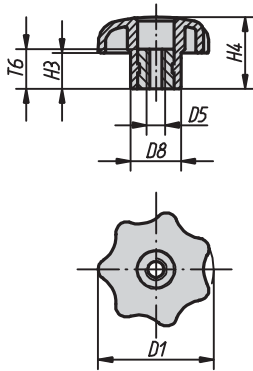
Form D mit Gewindebuchse ohne Deckel
