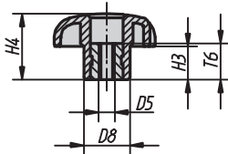
Form D mit Gewindebuchse ohne Deckel
