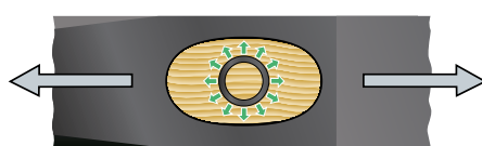
Der Ringkeil verteilt die Klemmkraft gleichmäßig auf 360°, also auch in Bewegungsrichtung. Die Faserstruktur des Holzes wird nicht zerstört. Der Hammerkopf lockert sich auch nach mehreren
