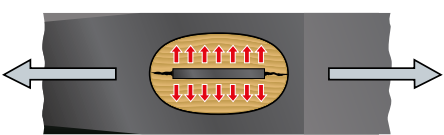
Der Flachkeil bringt keine Klemmkraft in Bewegungsrichtung auf.
